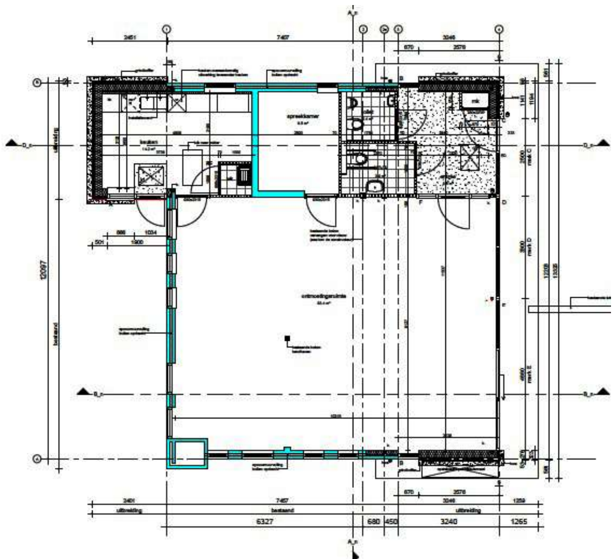
Plattegrond na verbouw.
